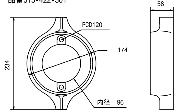
YS350 品番315-422-301
