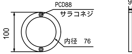
YS60/80 品番396-8257-400
