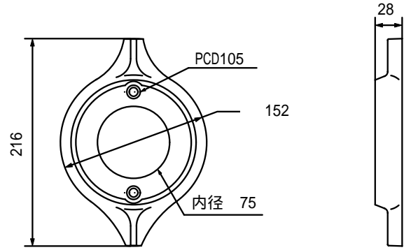
YS303 品番313-435-205
