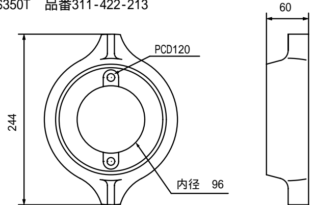
YS350T 品番311-422-213
