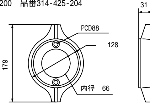
YS200 品番314-425-204
