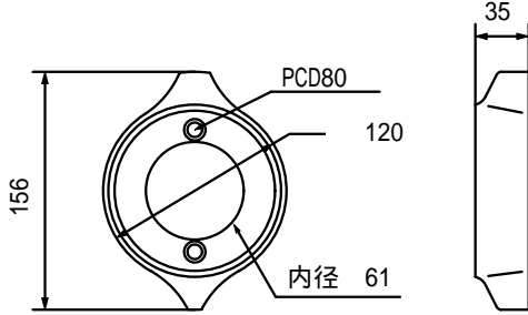
YS150/180 品番309-425-202
